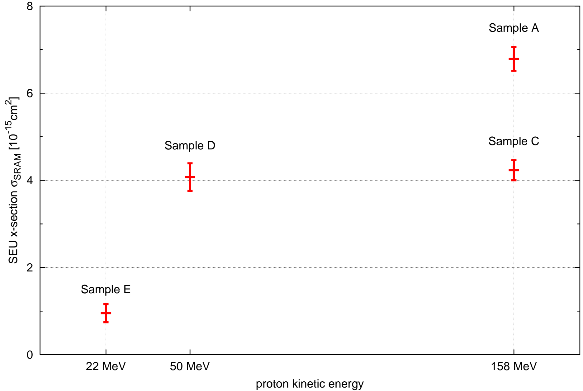
SEU Cross Section of the DSM SRAM cell
